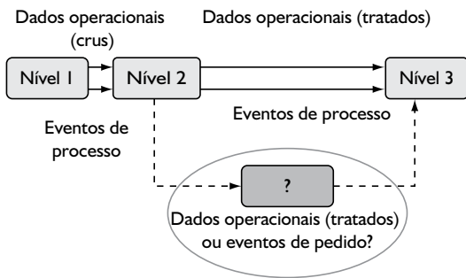
Figura 1. Arquitetura genérica de geração de eventos.
