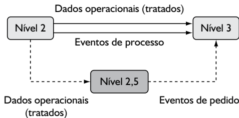
Figura 2. Arquitetura de geração de eventos baseado em sistema "standalone".
